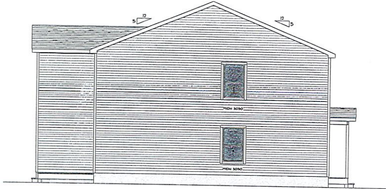
LEFT ELEVATION SCALE: 1/4" = 1'-0"
